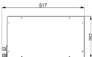
Unité intérieure vue de face :
